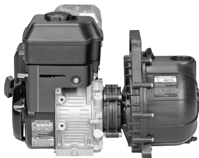
Impulsor con motor de gasolina dotado del sistema PROTEK
