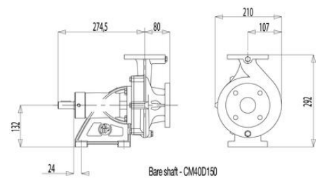
Bare shaft - CM40D150
