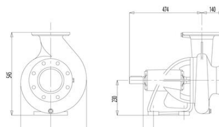
Bare shaft - CM125D225
