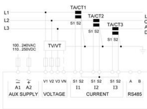
Innkobling, 3-fase uten N - måling med strømtransformatorer
