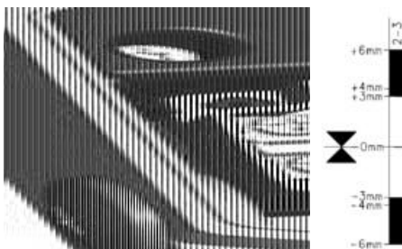
Linespenn sensor som gir signal ved endring på \pm 3 mm. Nødstopp ved \pm 4 mm.
