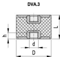
DVA.3 - 8 - 8 - M3 - 55 D L d I Shore A
