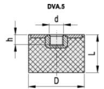
DVA.5 - 10 - 10 - M4 - 55 D L d I Shore A
