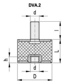
DVA.2 - 8 - 8 - M3 - 6 - 55 D L d I Shore A
