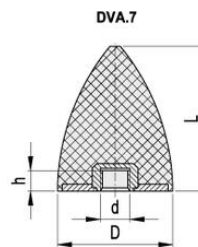
DVA.7 - 20 - 24 - M6 - 55 D L d I Shore A
