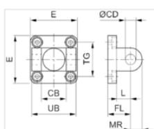
Dimensjoner
